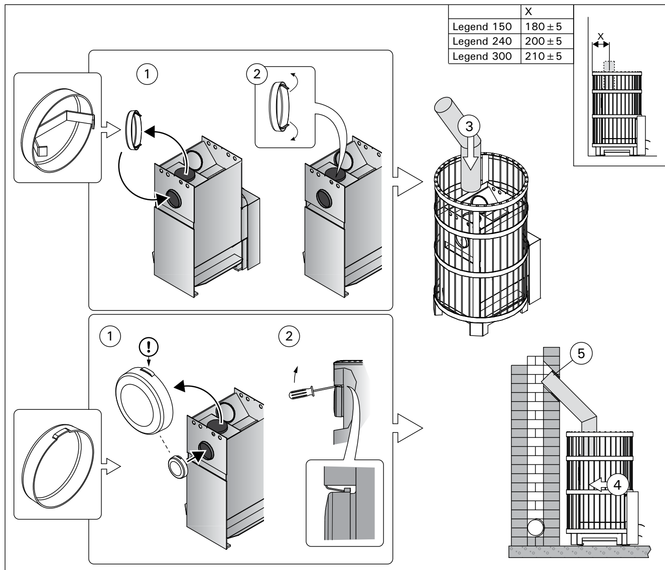
Kuva 12. Kiukaan liittäminen muurattuun savuhormiin yläliitännäaukon kautta (mitat millimetreinä)
