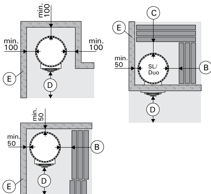
Рисунок 9. Безопасные расстояния (все размеры приведены в миллиметрах)
