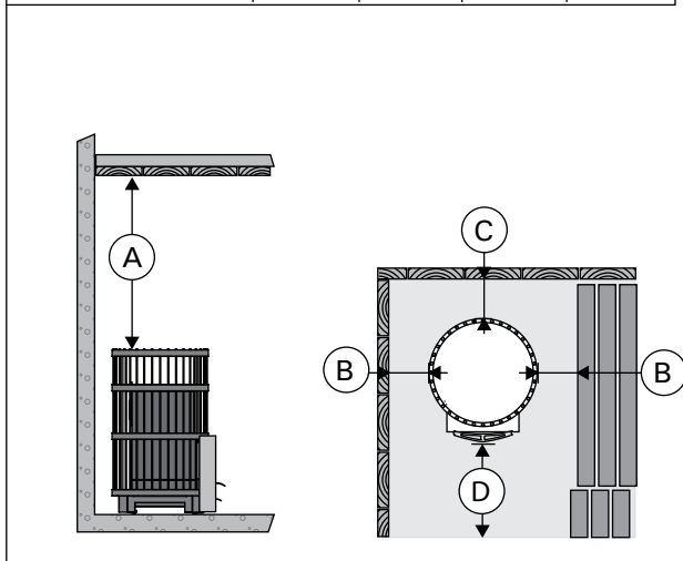
Рисунок 9. Безопасные расстояния (все размеры приведены в миллиметрах)
