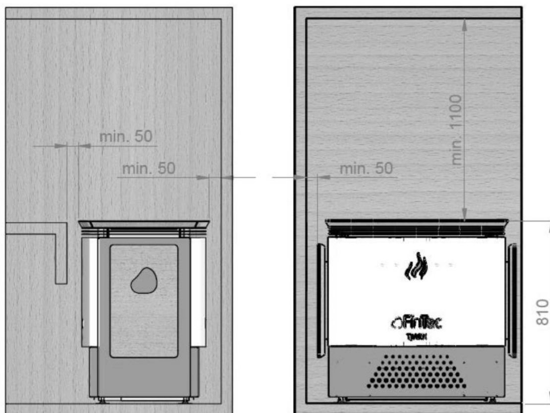
Abbildung 4: Sicherheitsabstände
