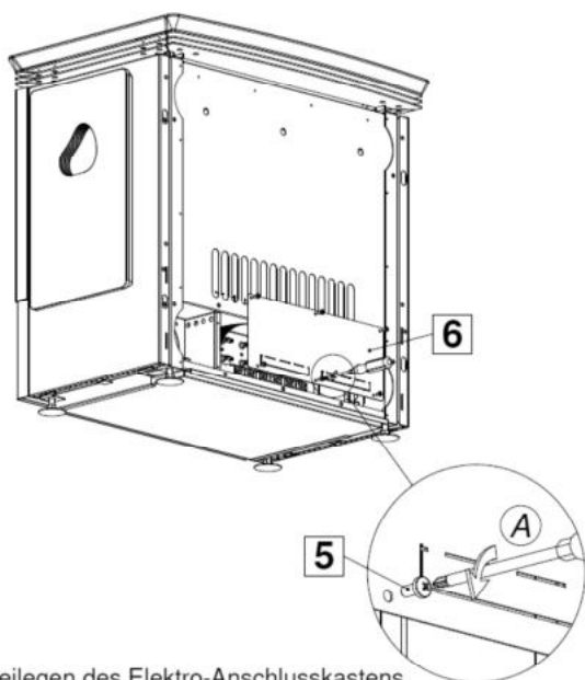
Freilegen des Elektro-Anschlusskastens
