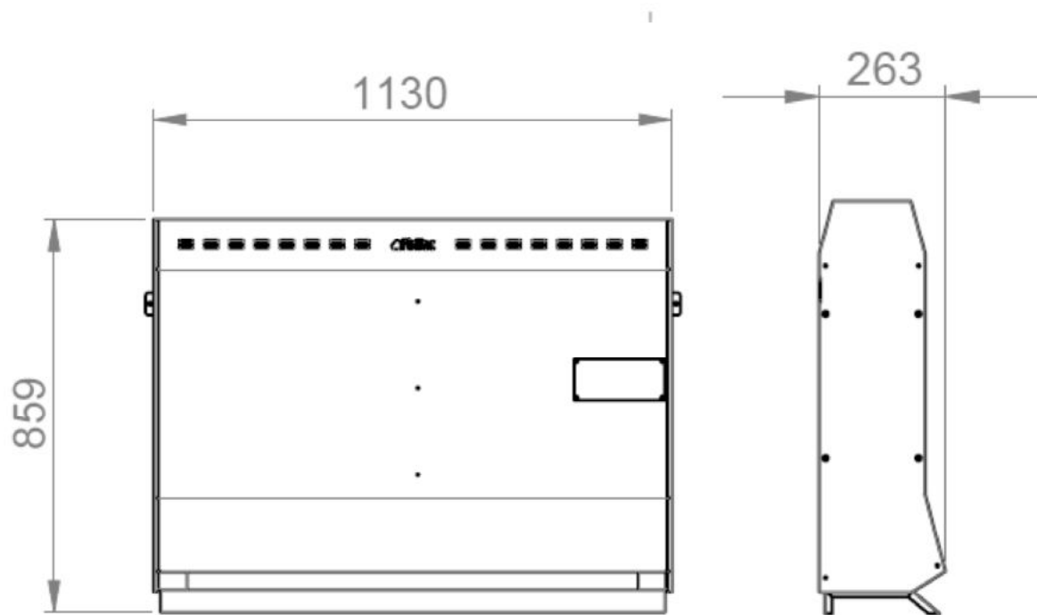
Abbildung 2: Saunaofen
