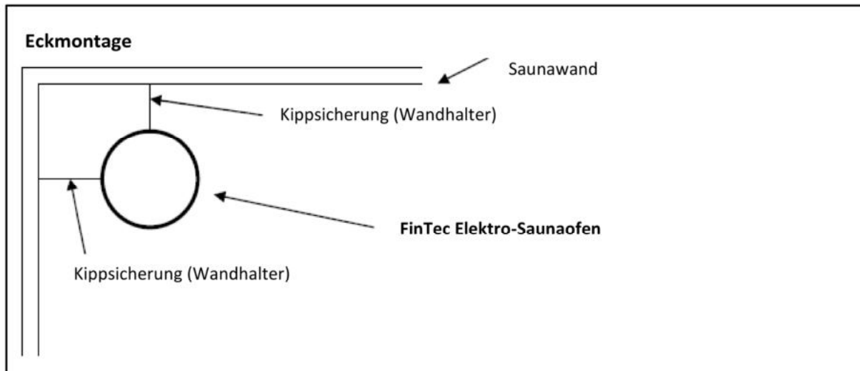
Abbildung 4: Schema Eckmontage
