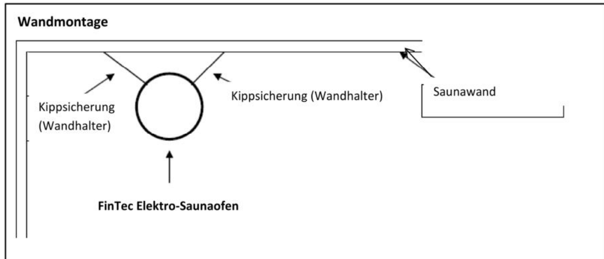
Abbildung 5: Schema Wandmontage
